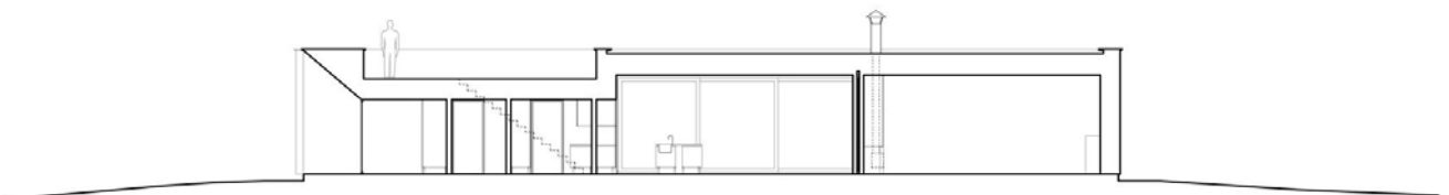
Corte Transversal
